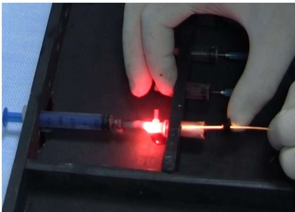
Рисунок 7. Моделирование ЭВЛО в сегменте вены на стенде.
