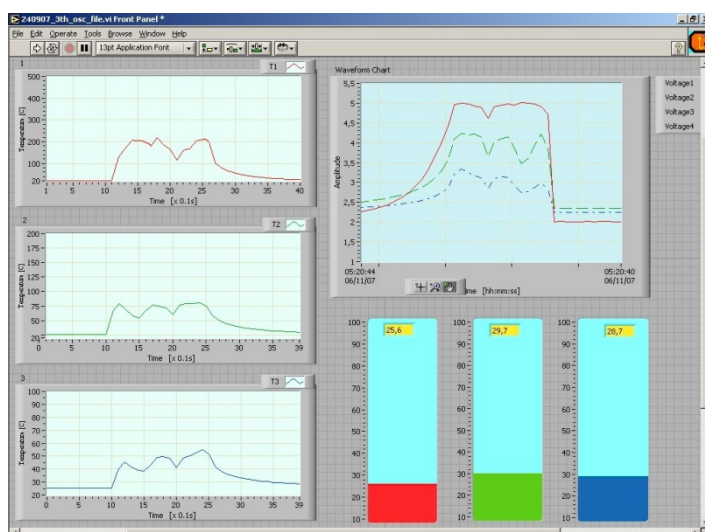
Рисунок 2. Графический интерфейс программного обеспечения для регистрации и контроля в реальном времени показаний термодатчиков.
