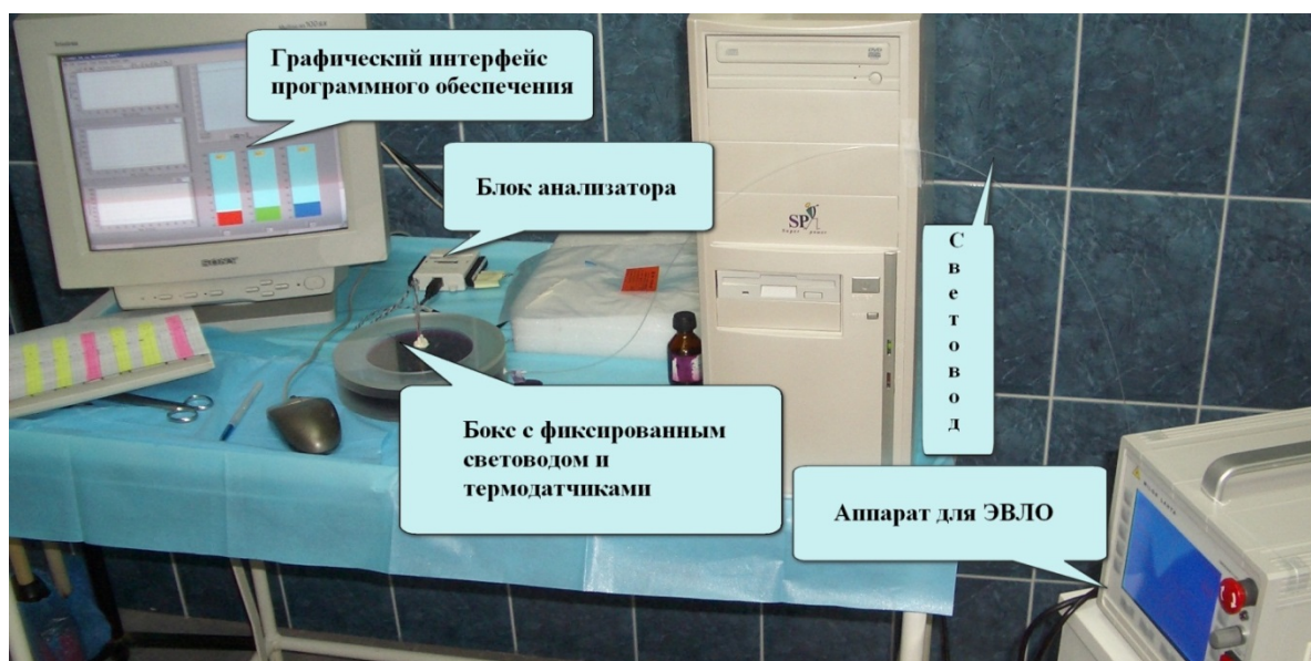
Рисунок. 1. Экспериментальный стенд для определения температуры при проведении эндовазальной лазерной облитерации на различных расстояниях от рабочей части световода in vitro .
