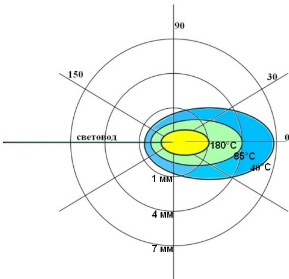
Рисунок 9. Изотермы 40°C, 85°C, 180°C при моделировании ЭВЛО в режиме: 1470 нм. Мощность 15 Вт, импульс 900 мс, интервал между импульсами 100 мс. Энергия импульса 13.5 Дж.
