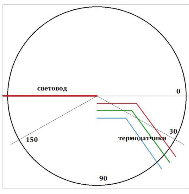
Рисунок 4. Схема экспериментальной установки для определения температуры на различных расстояниях от рабочей части световода при проведении эндовазальной лазерной облитерации in vitro (вид сверху, датчики расположены со смещением 90 относительно оси световода).
